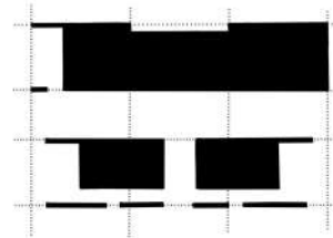
ROZOHRAŤIE HMOTY POMOCOU TIENIACÝCH STIEN
