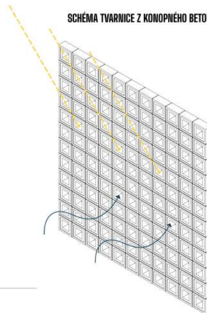
KONOMETRIA PERFOROVANÁ EXTERIÉROVÁ STĚNA - TIENENIE, DEFINOVANIE PROSTORU
